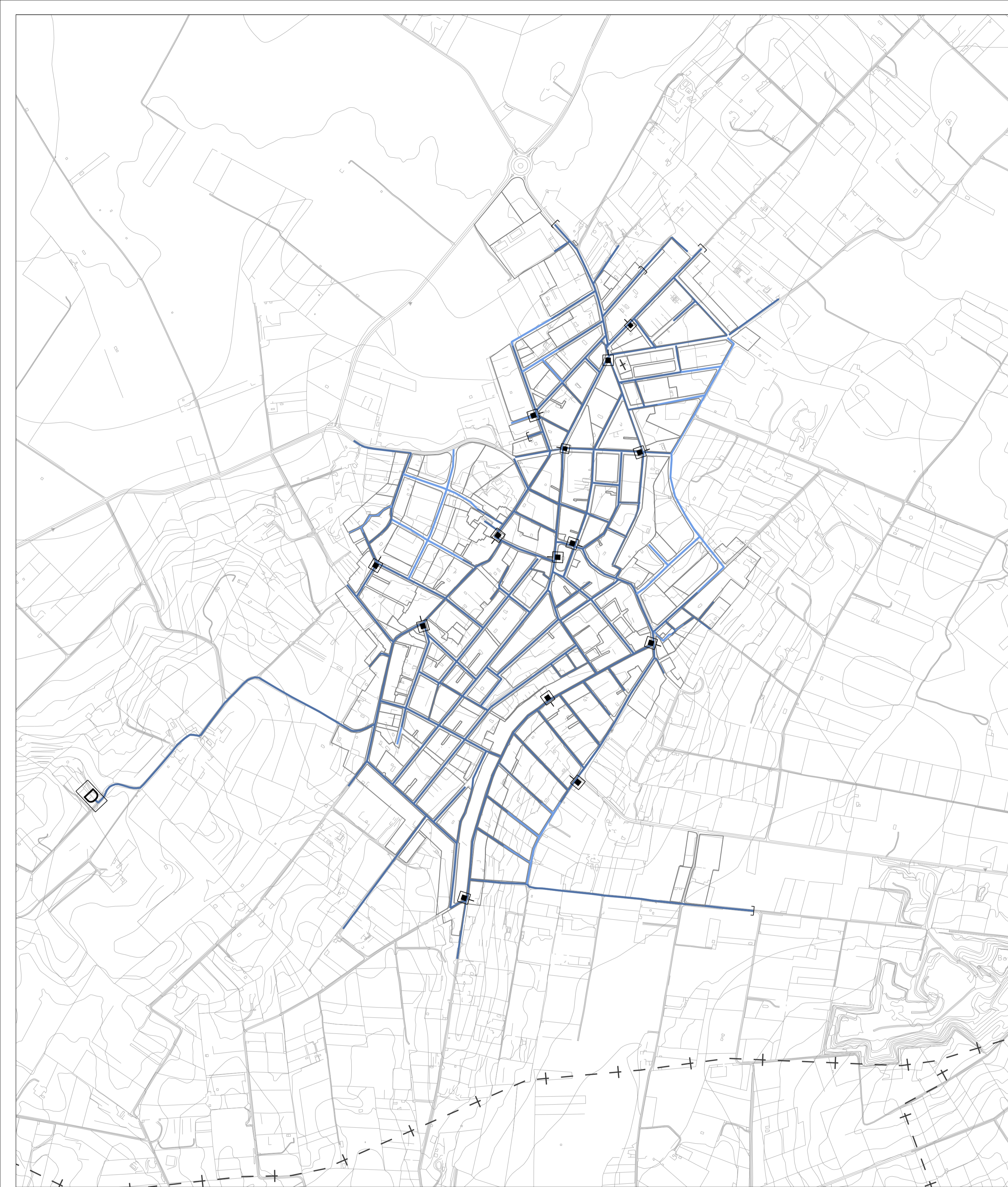
XARXA D'AIGUA POTABLE
