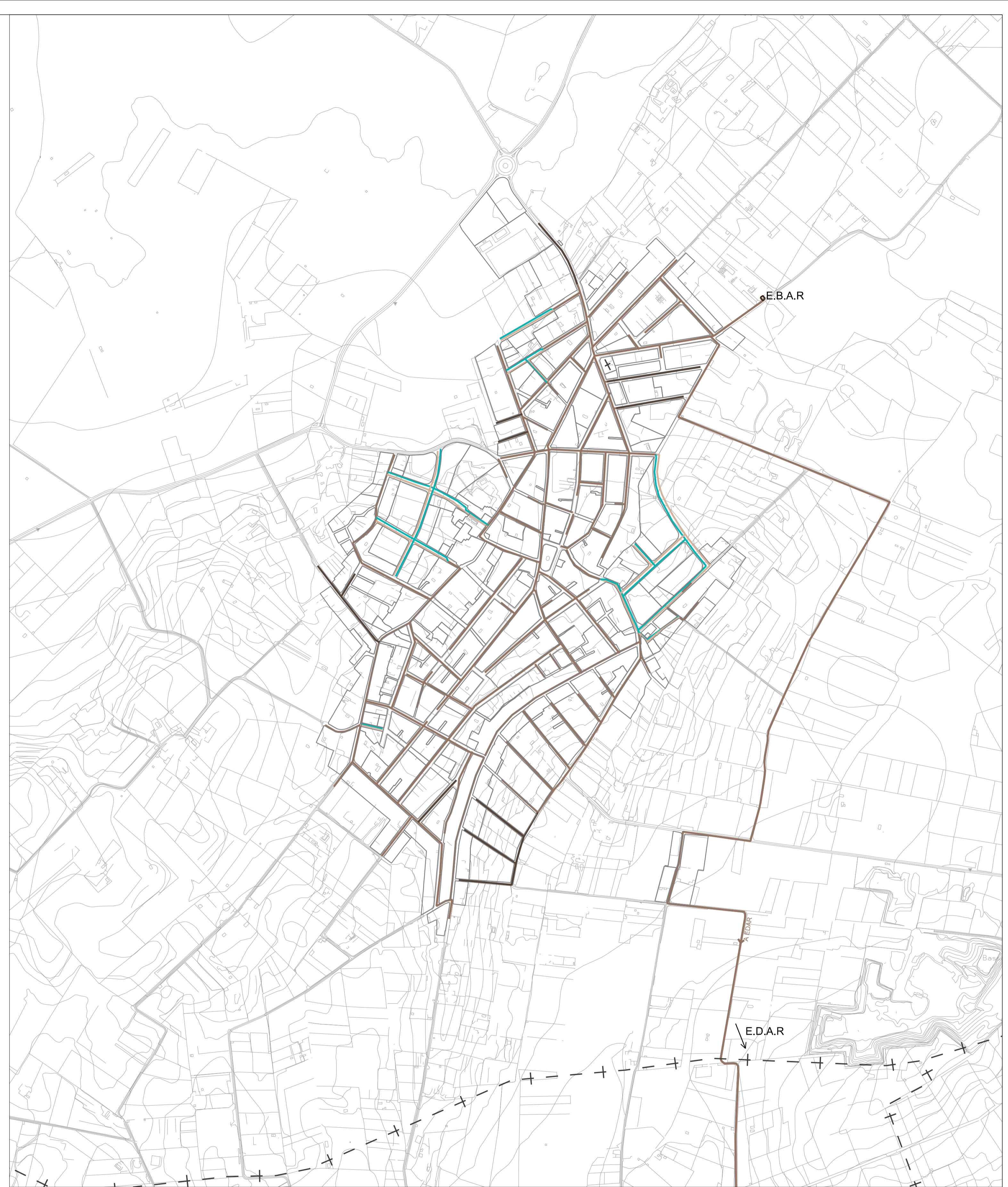
XARXA DE CLAVEGUERAM
